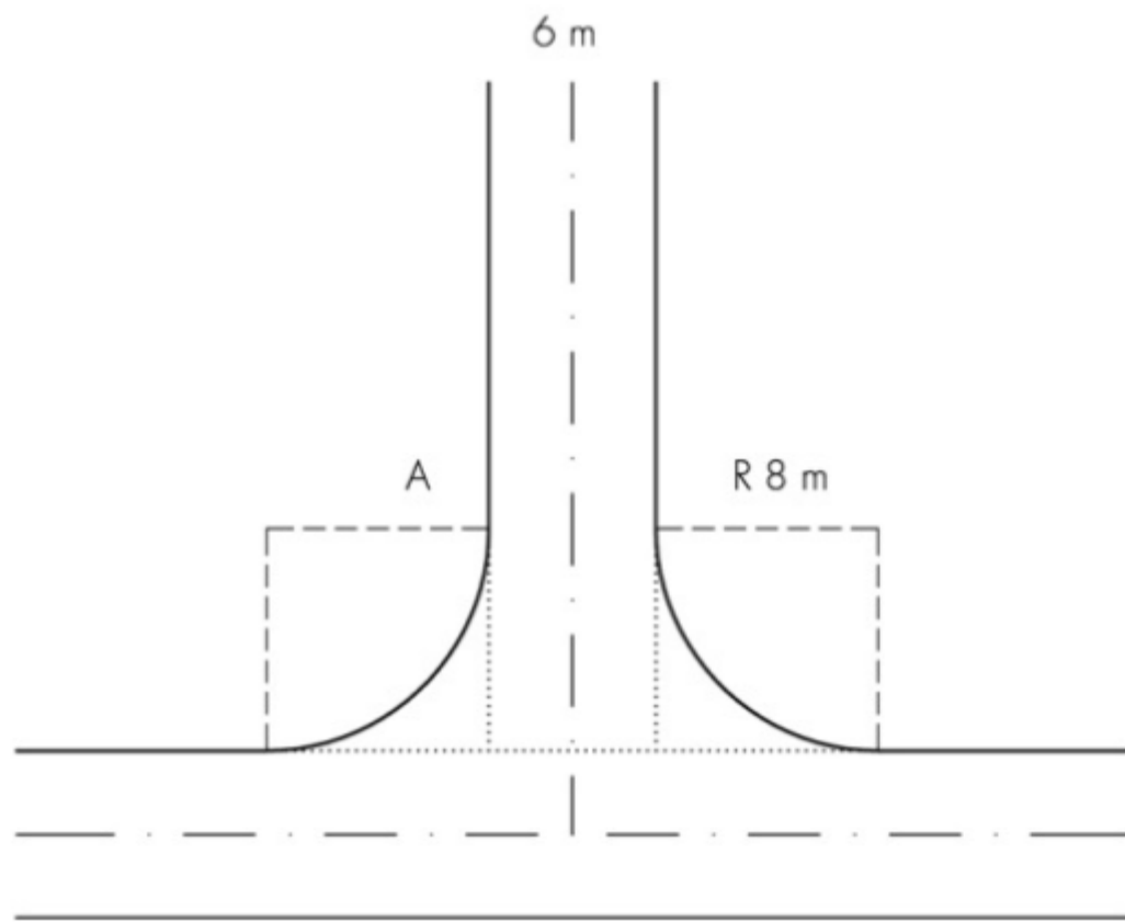
Obr. 6.35 Pripojovacie polomery cestných križovatiek
