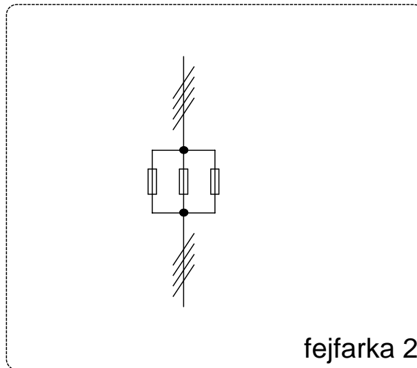
schema 1pólové "pojistková skříň"
